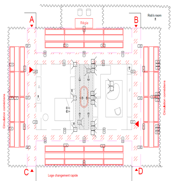
1 : Plan de scénographie avec l'éclairage. © Manuel Desfeux
