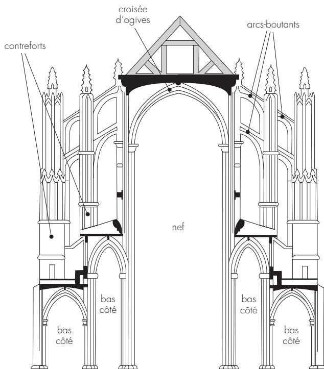
Coupe d'une église gothique.
